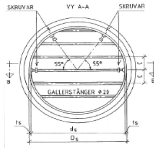
Skiss/ritningsförslag
