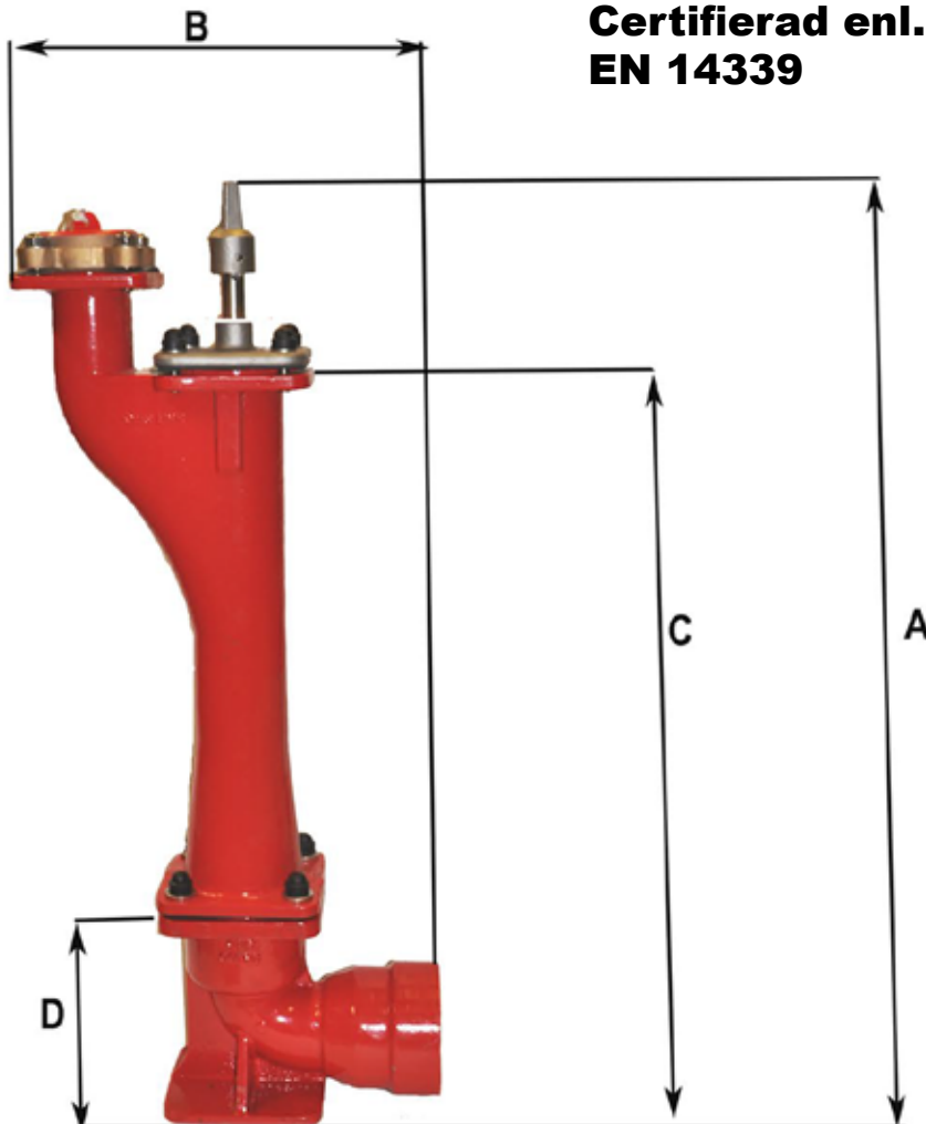
Byggmått
