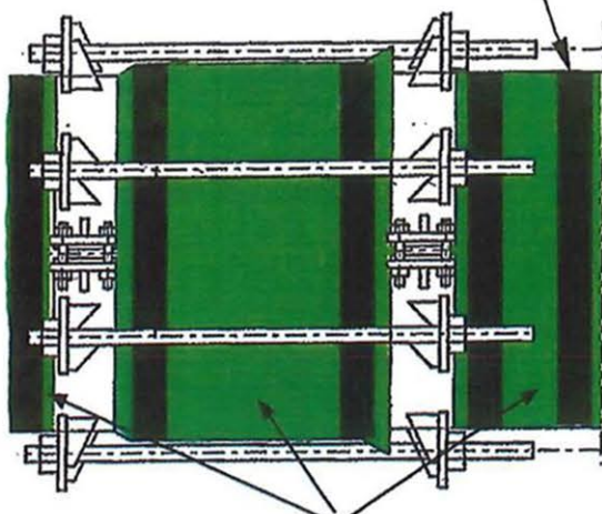
Gummiringsfogade stålrör
