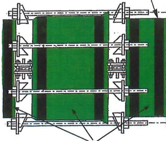
Gummiringfogade stålrör
