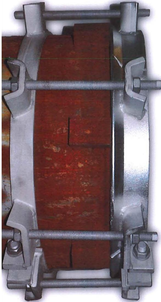
Gummiringfogade stålrör
